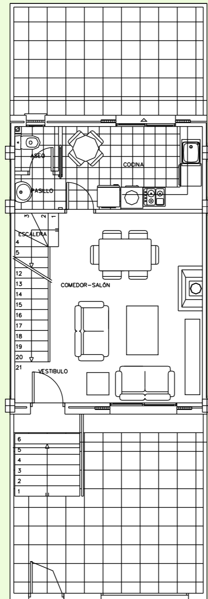
PLANTA BAJA
