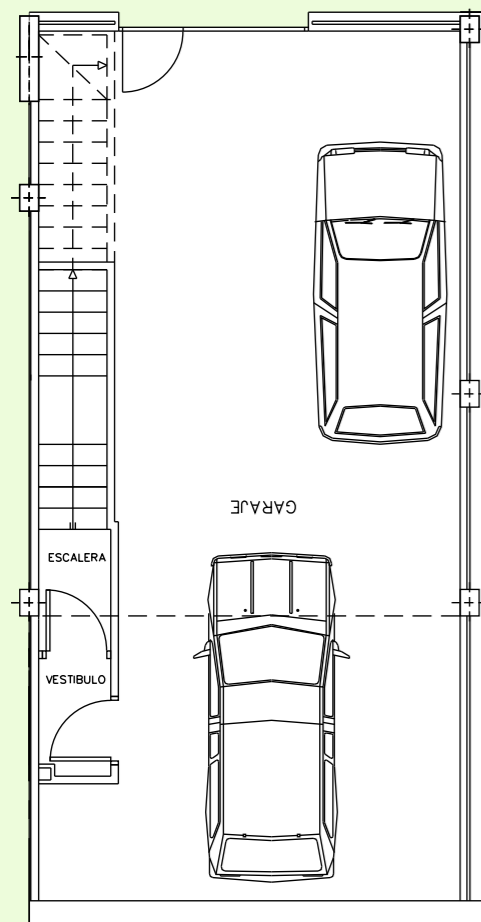
PLANTA SOTANO
